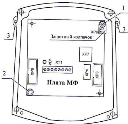
Рисунок 1 - Места пломбирования преобразователей и нанесения знака поверки
