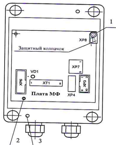
Рисунок 2- Места пломбирования преобразователей и нанесения знака поверки
