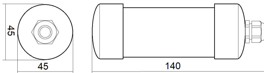
Рисунок 3.1 – Габаритные размеры Модуля
